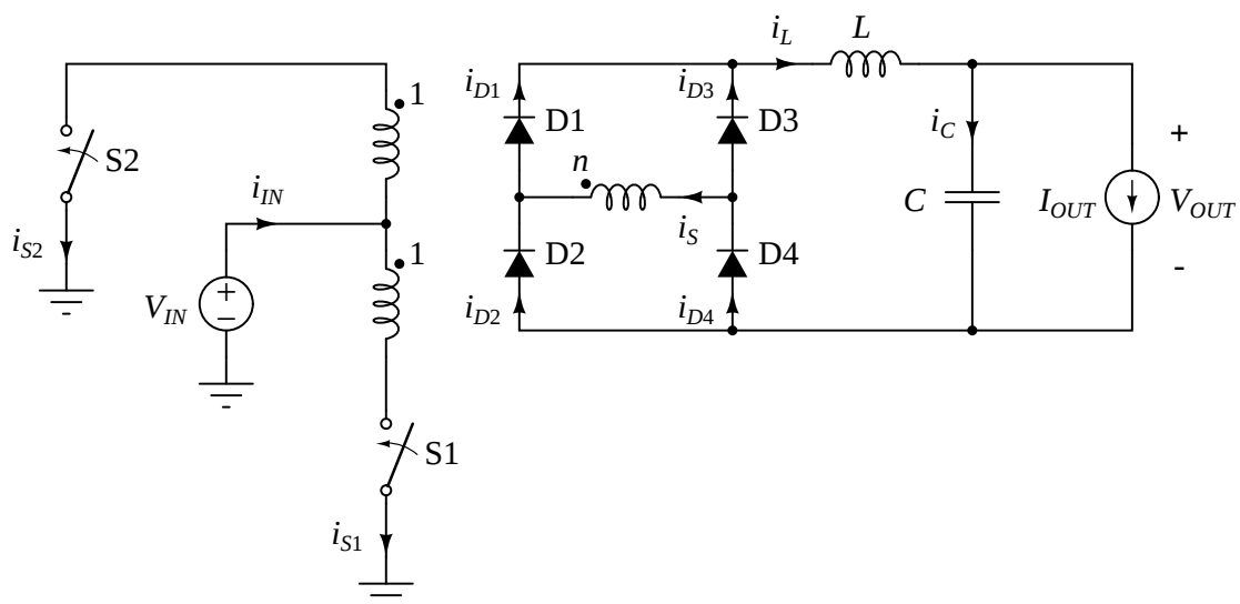
Slika 3: Push-pull konvertor sa Grecovim spojem na izlazu.
