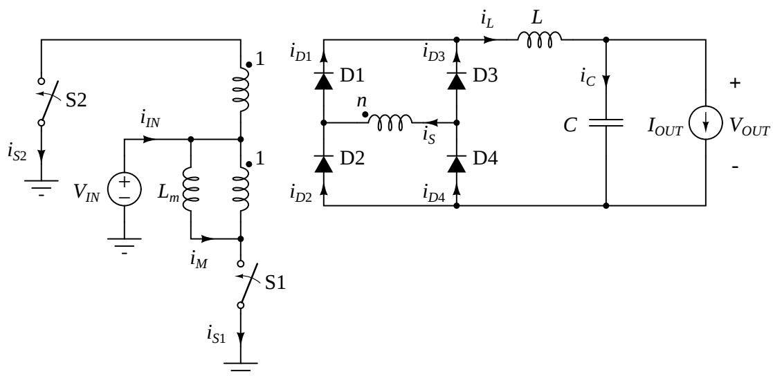
Slika 4: Push-pull konvertor sa Grecovim spojem na izlazu, izdvojena magnetizaciona induktivnost.
