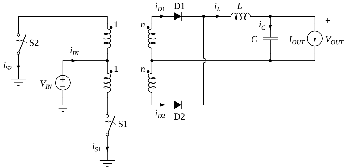
Slika 1: Push-pull konvertor.
