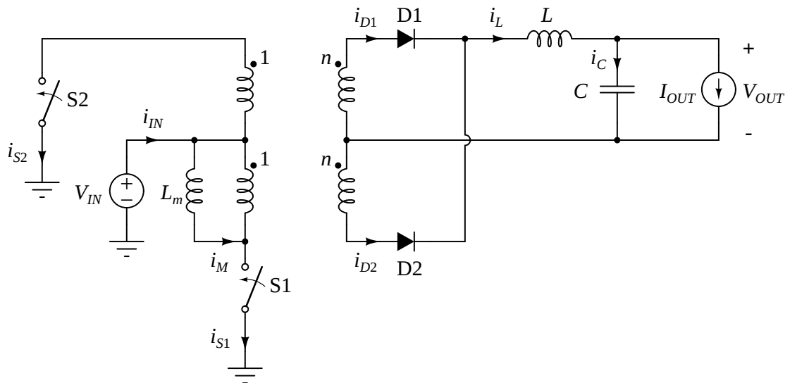
Slika 2: Push-pull konvertor, izdvojena magnetizaciona induktivnost.
