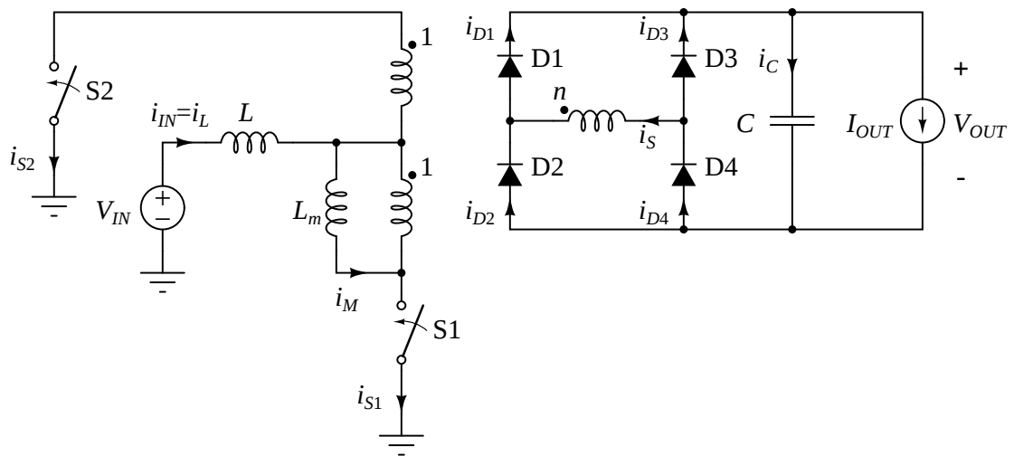
Slika 4: Izolovani boost konvertor sa Grecovim spojem na izlazu, izdvojena magnetizaciona induktivnost.
