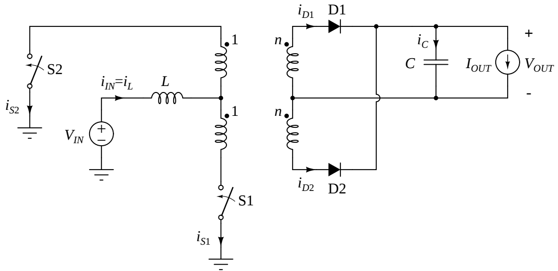
Slika 1: Izolovani boost konvertor.
