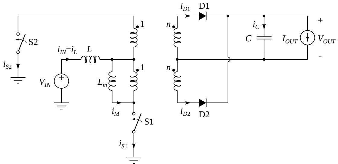
Slika 2: Izolovani boost konvertor konvertor, izdvojena magnetizacijska induktivnost.
