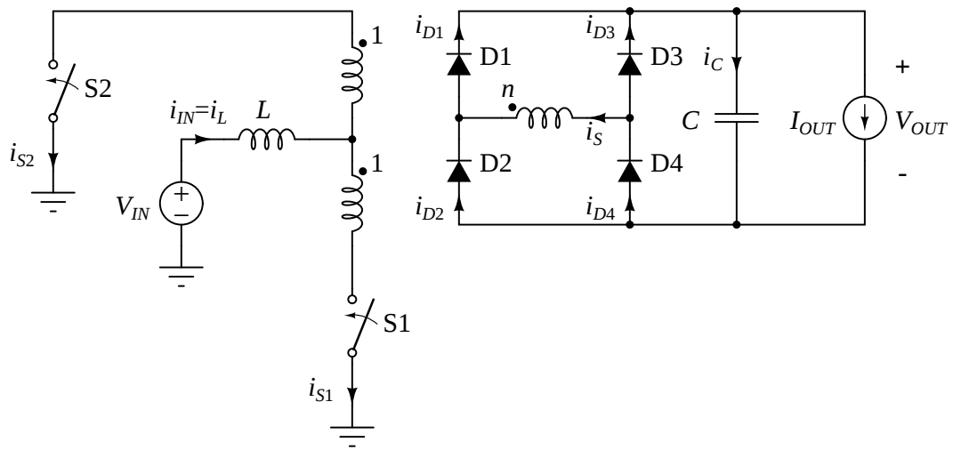
Slika 3: Izolovani boost konvertor sa Grecovim spojem na izlazu.
