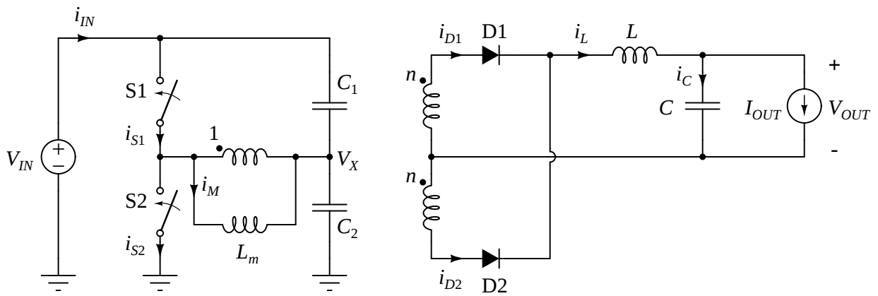
Slika 2: Half-bridge konvertor, izdvojena magnetizacijska induktivnost.
