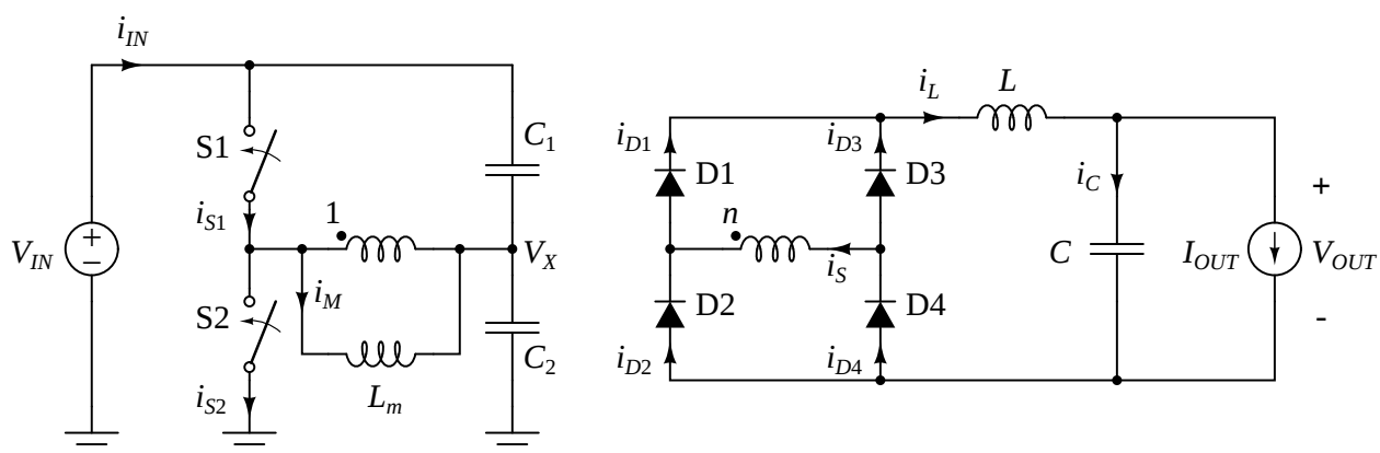
Slika 4: Half-bridge konvertor sa Grecovim spojem na izlazu, izdvojena magnetizaciona induktivnost.
