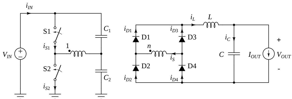
Slika 3: Half-bridge konvertor sa Grecovim spojem na izlazu.
