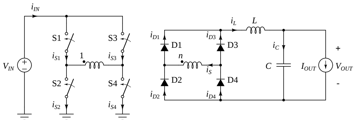
Slika 3: Full-bridge konvertor sa Grecovim spojem na izlazu.
