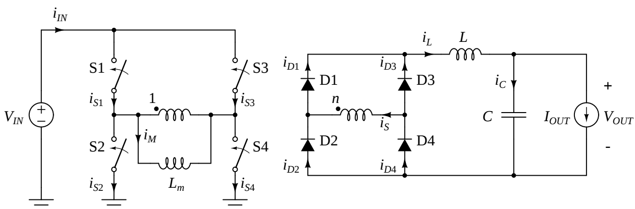
Slika 4: Full-bridge konvertor sa Grecovim spojem na izlazu, izdvojena magnetizaciona induktivnost.
