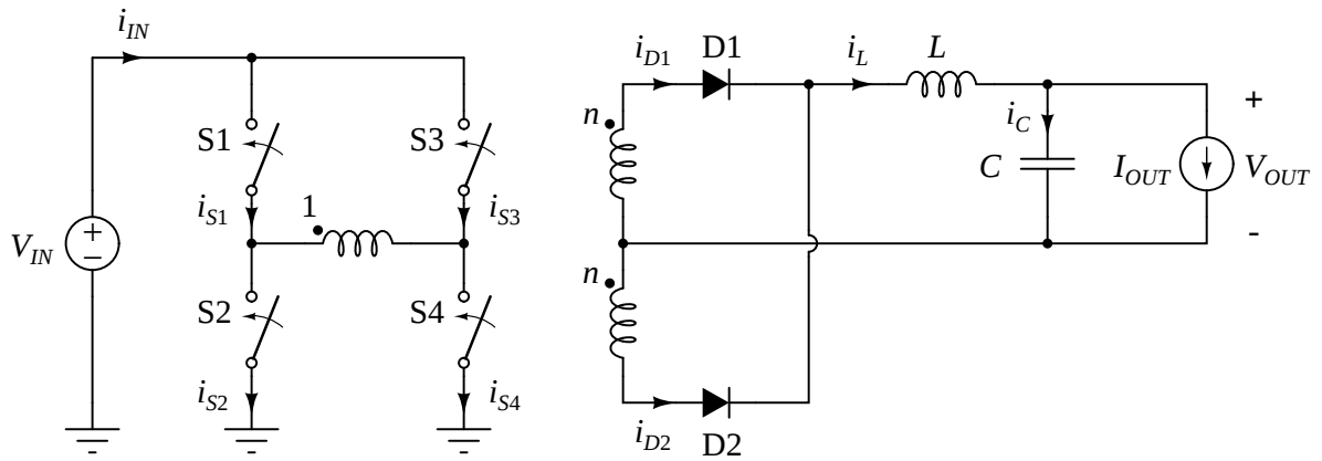
Slika 1: Full-bridge konvertor.
