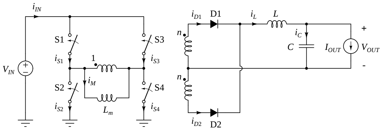
Slika 2: Full-bridge konvertor, izdvojena magnetizaciona induktivnost.
