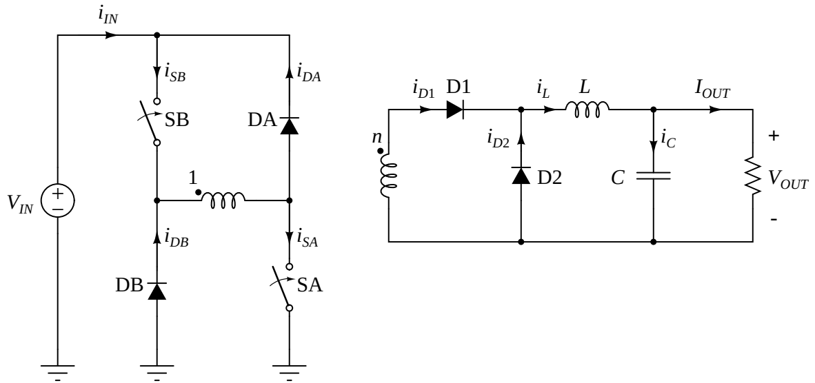
Slika 3: Forward konvertor sa dva prekidača.
