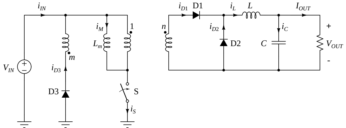
Slika 2: Forward konvertor, izdvojena magnetizaciona induktivnost.
