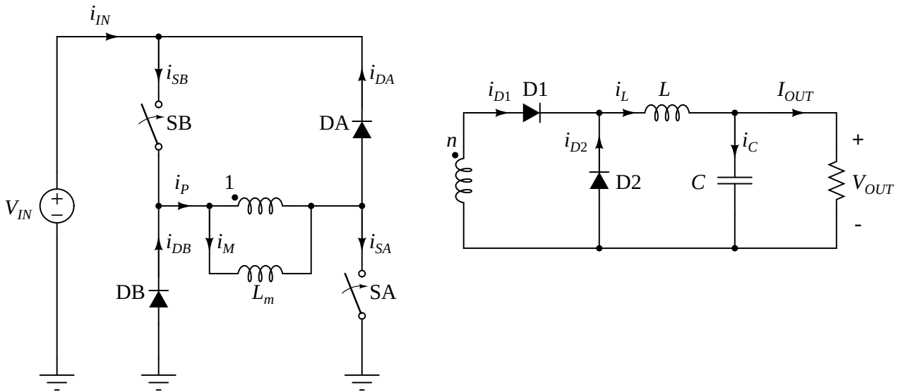
Slika 4: Forward konvertor sa dva prekidača, izdvojena magnetizaciona induktivnost.
