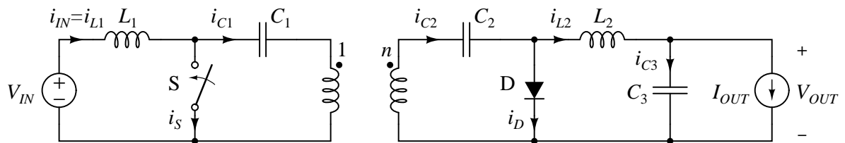
Slika 3: Ćukov konvertor sa galvanskim razdvajanjem.
