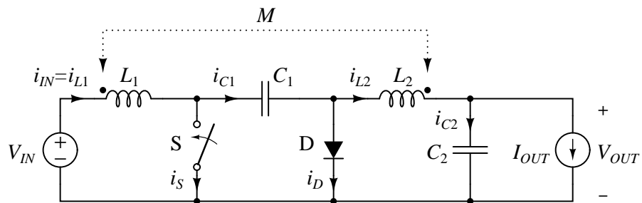
Slika 2: Ćukov konvertor sa magnetnom spregom između kalemova.
