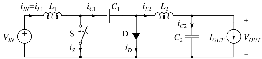
Slika 1: Ćukov konvertor.
