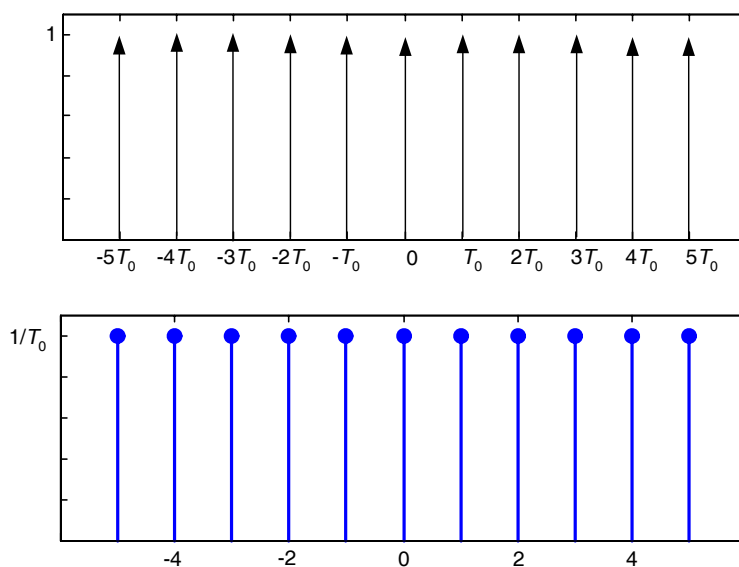
Periodični impulsni signal \text{comb}(t) i njegovi Furijeovi koeficijenti
