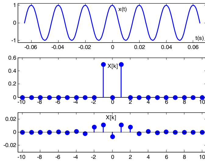
Kosinusna funkcija i njeni Furijeovi koeficijenti za dve vrednosti intervala razvoja: T_{F1}=T_{ox} i T_{F1}=1.5T_{ox}
