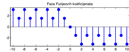
Modifikovana periodična povorka pravougaonih impulsa i koeficijenti njenog razvoja u Furijeov red
