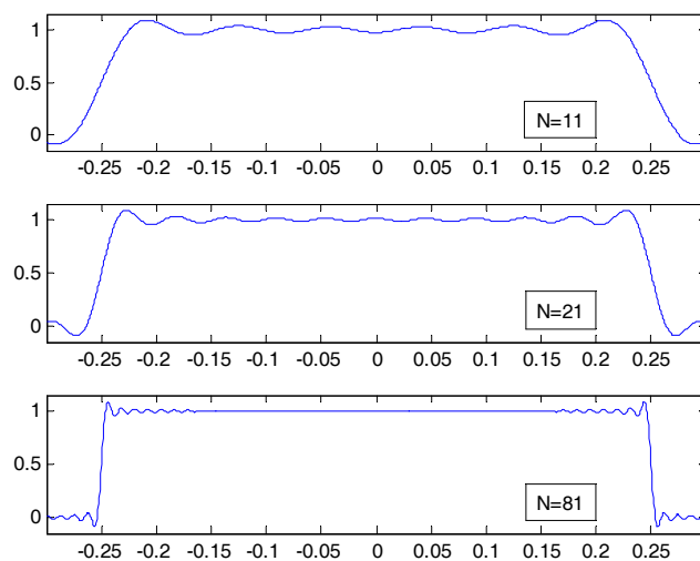
Konvergencija razvoja periodične povorka pravougaonih impulsa u Furijeov red
