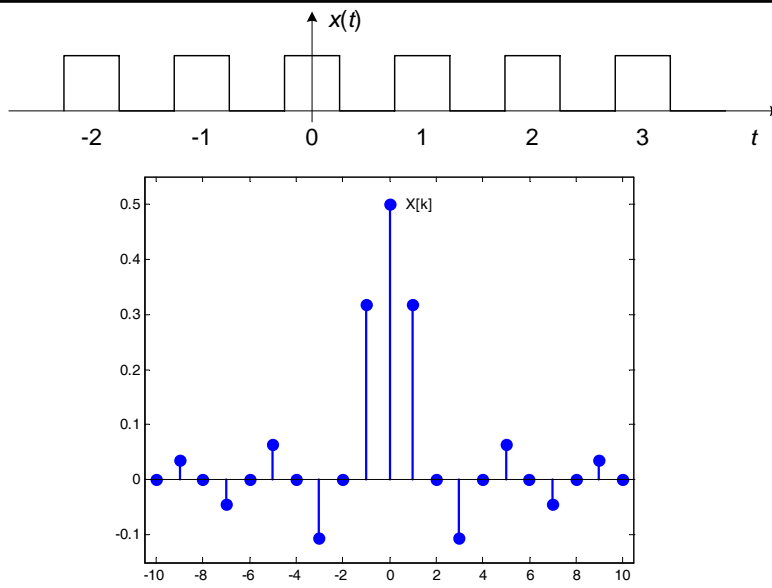
Periodična povorka pravougaonih impulsa i koeficijenti njenog razvoja u Furijeov red
