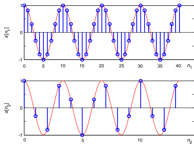
Dve diskretne sinusoide dobijene odabiranjem iste vremenski kontinualne sinusoide
