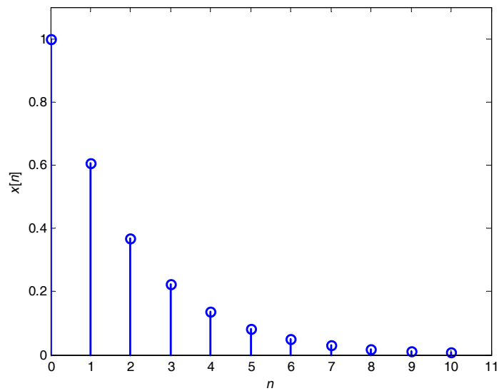
Primer diskretne eksponencijalne funkcije
