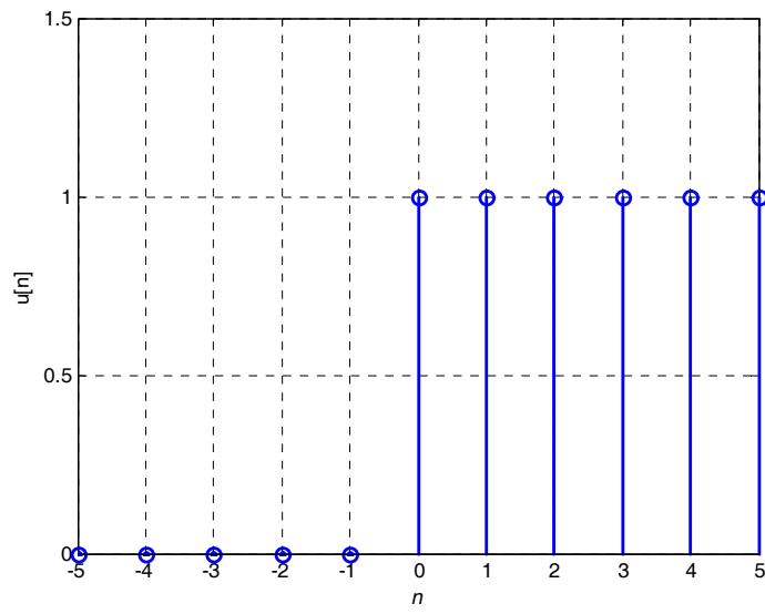
Diskretni jedinični niz
