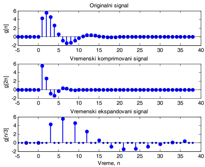
Skaliranje vremenske ose: (a) Kompresija, K = 2 , (b), Ekspanzija, K = 3
