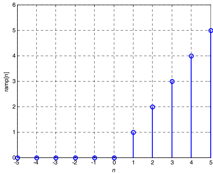
Diskretni linearni niz
