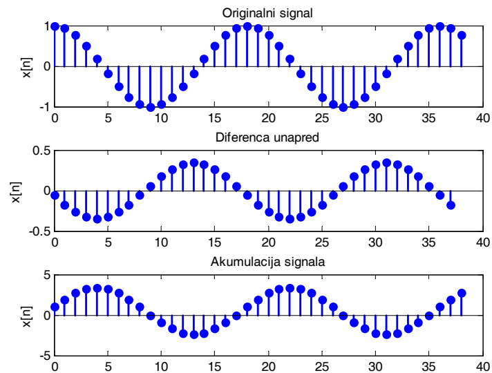
Prva diferencija i akumulacija diskretne vremenske funkcije
