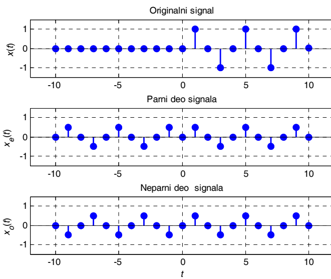
Primer rastavljanja diskretnog signala na parni i neparni deo
