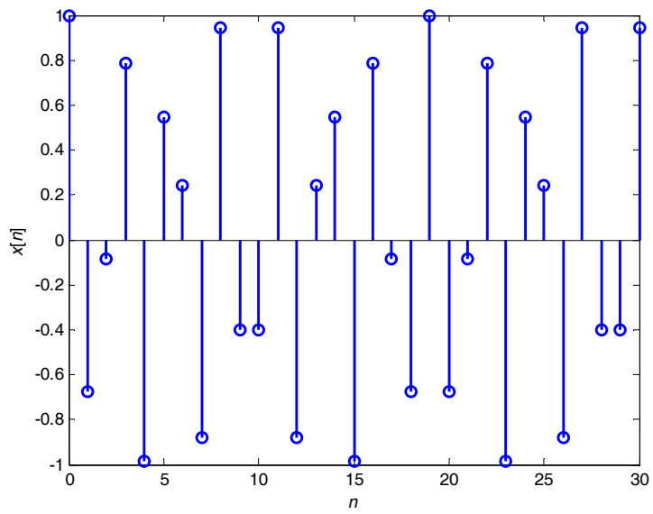
Primer diskretne sinusoide koja po obliku ne podseća na sinusoidu
