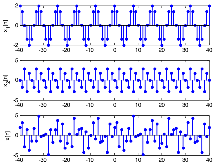
Primer složenog diskretnog periodičnog signala
