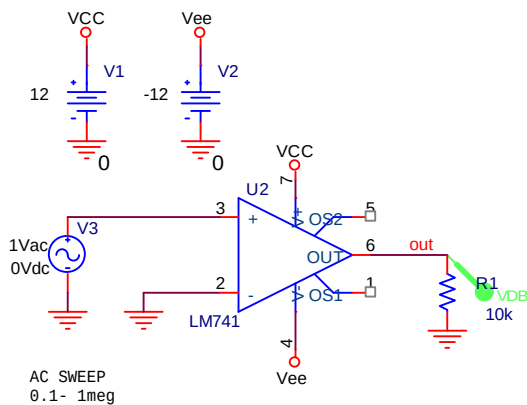
AC Sweep – Frekvencijske karakteristike
